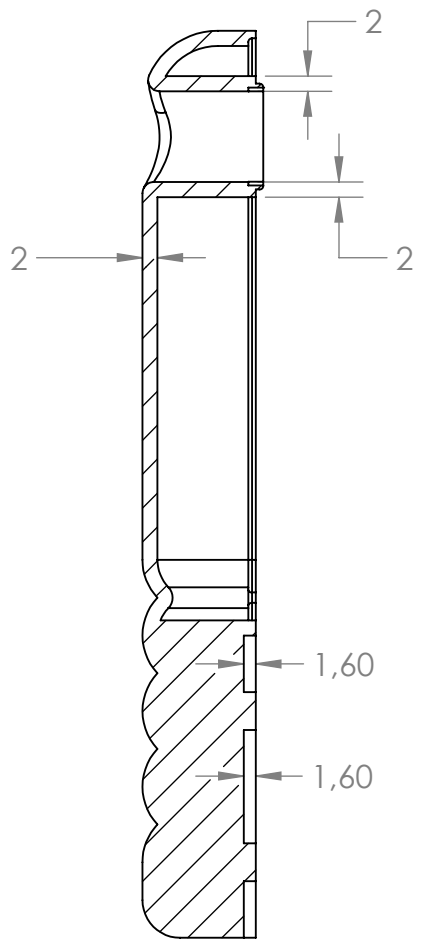
COUPE A-A
